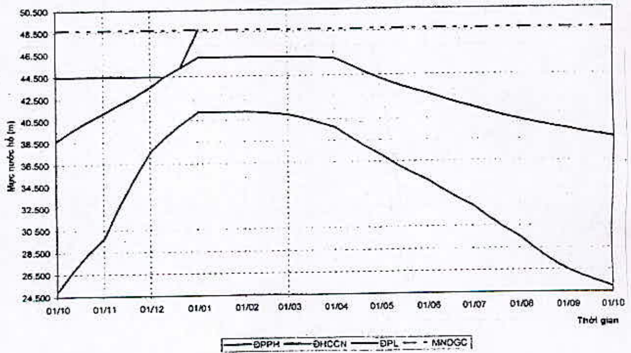
BIỂU ĐỒ ĐIỀU PHỐI HỒ NÚI MỘT
