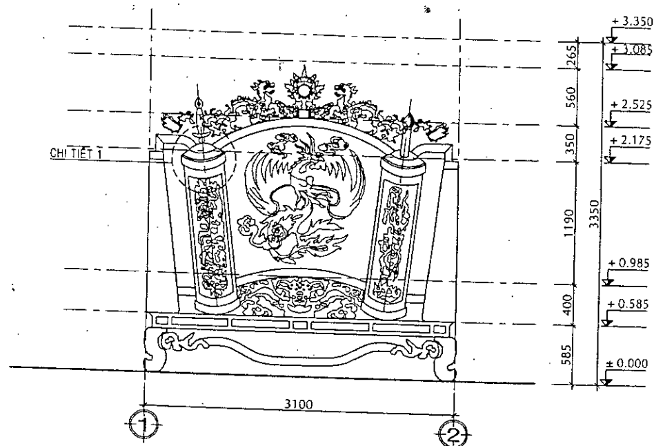
MẶT ĐỨNG TRỤC 1-2, TL:1/50
