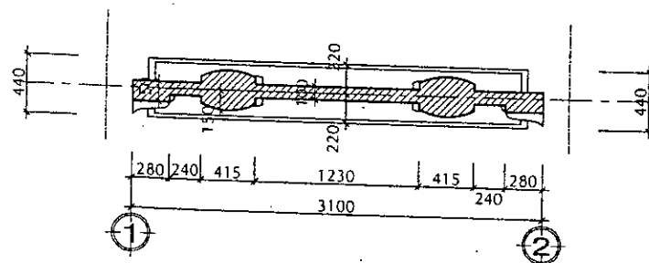
MẶT BẰNG BỨC BÌNH PHONG, TL:1/50
