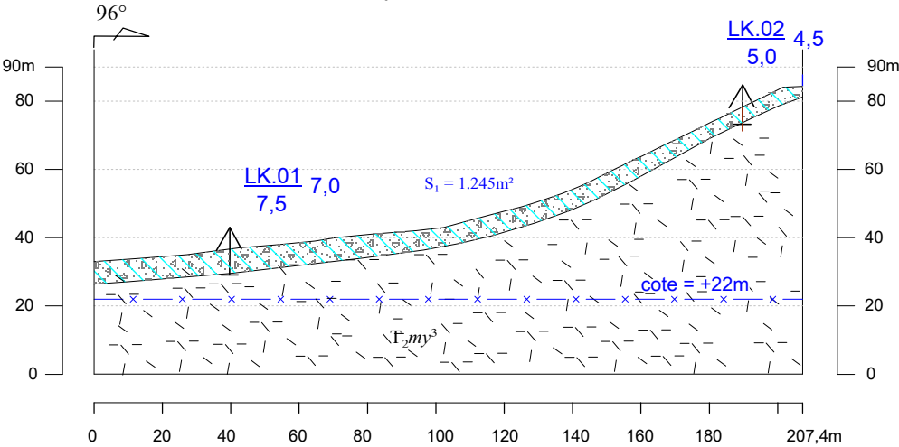
MẶT CẮT TÍNH TRỮ LƯỢNG - TUYẾN T1-1
