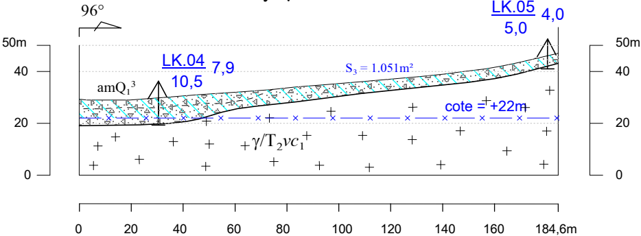
MẶT CẮT TÍNH TRỮ LƯỢNG - TUYẾN T2
