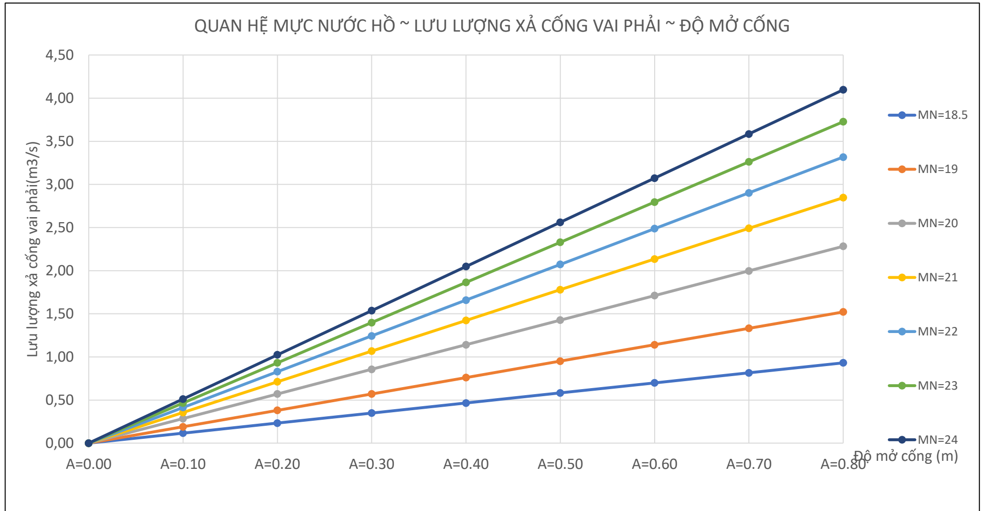
Hình PL5.2: Biểu đồ quan hệ lưu lượng Q và độ mở cửa cống a và mực nước hồ Z (Cống vai phải)
