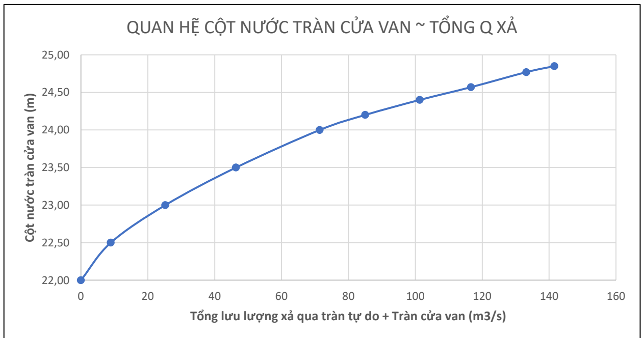
Hình PL 6.3: Biểu đồ quan hệ tổng lưu lượng Q xả tràn và mực nước hồ Z
