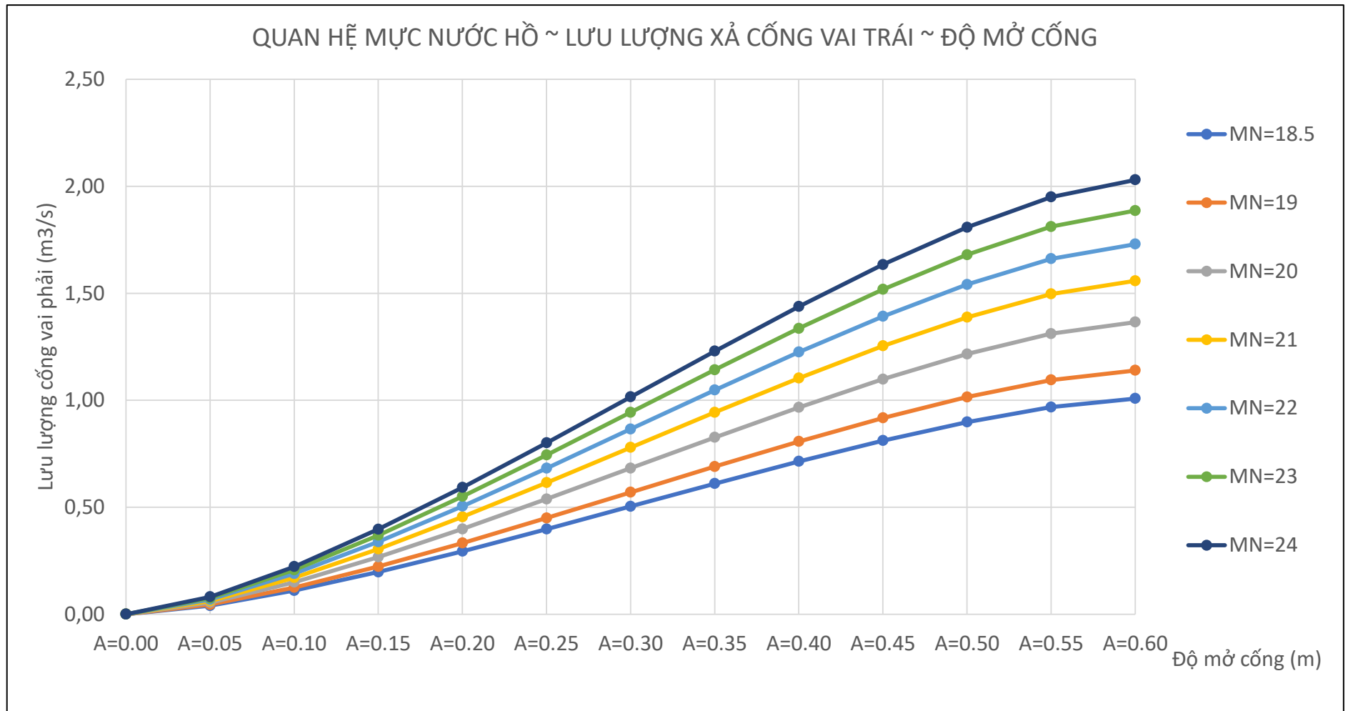
Hình PL5.1: Biểu đồ quan hệ lưu lượng Q và độ mở cửa cống a và mực nước hồ Z(Cống vai trái)
