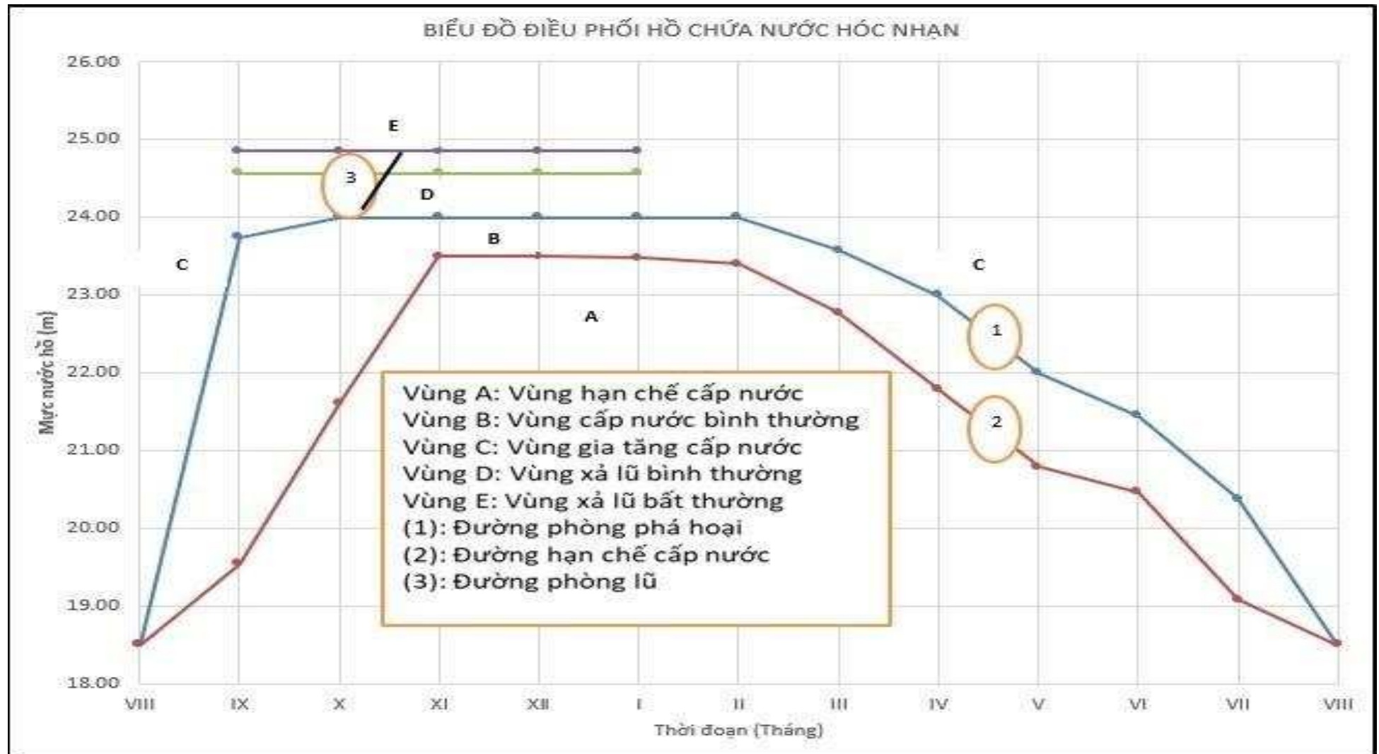
Hình PL7.1 Biểu đồ điều phối hồ chứa nước Hóc Nhạn
