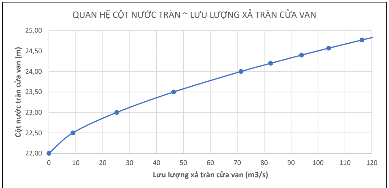
Hình PL 6.2: Biểu đồ quan hệ lưu lượng Q xả tràn có cửa và mực nước hồ Z
