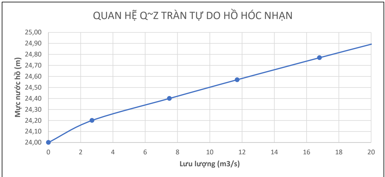
Hình PL 6.1: Biểu đồ quan hệ lưu lượng Q xả tràn tự do và mực nước hồ Z
