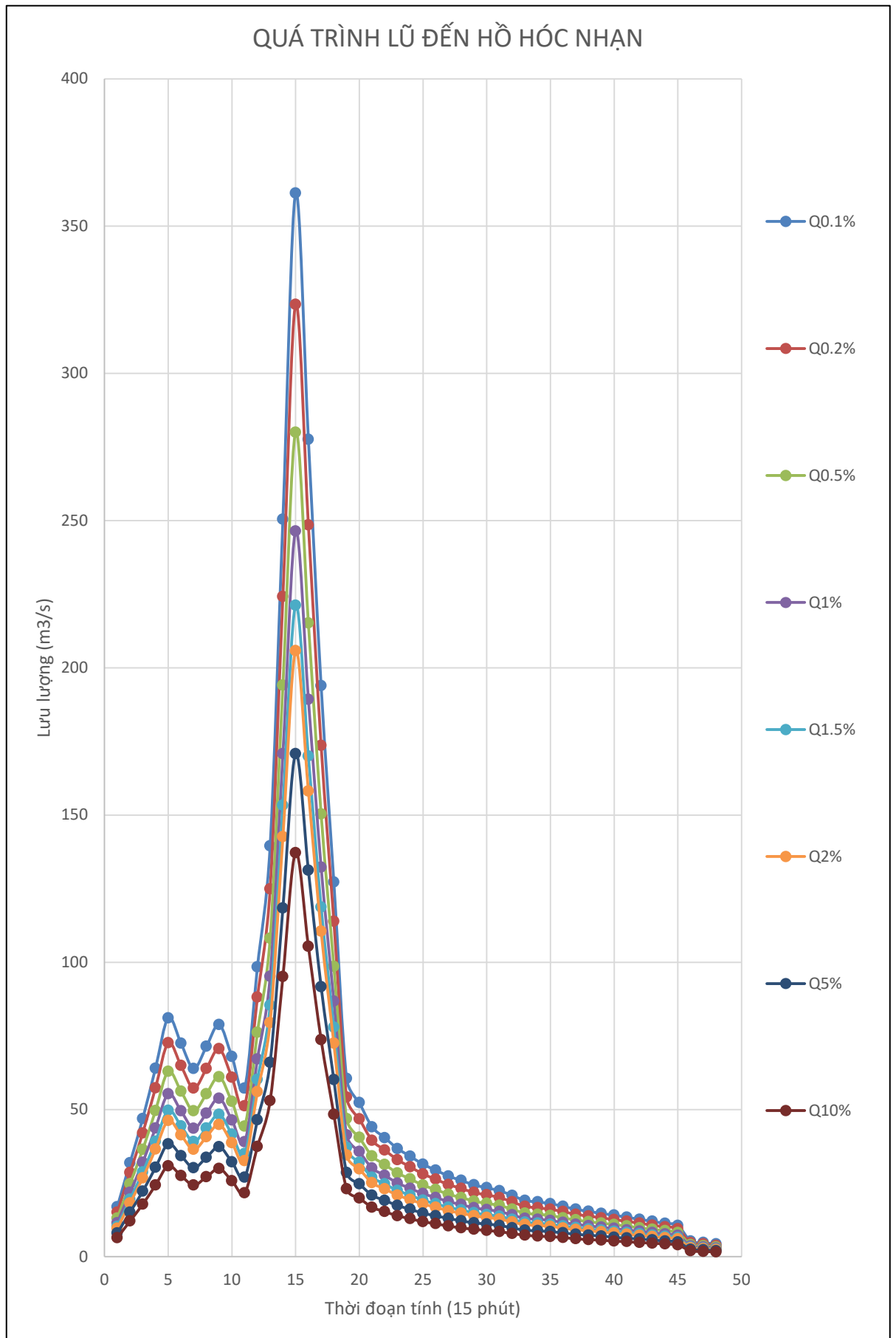
Hình PL 2.2: Đường quá trình lũ thiết kế hồ Hóc Nhạn
