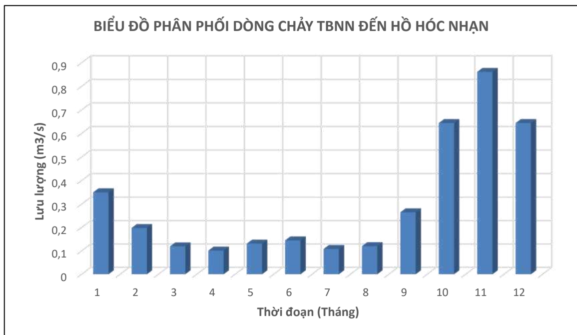
Hình PL 2.1: Biểu đồ phân phối dòng chảy TBNN đến hồ Hóc Nhạn (m 3 /s)
