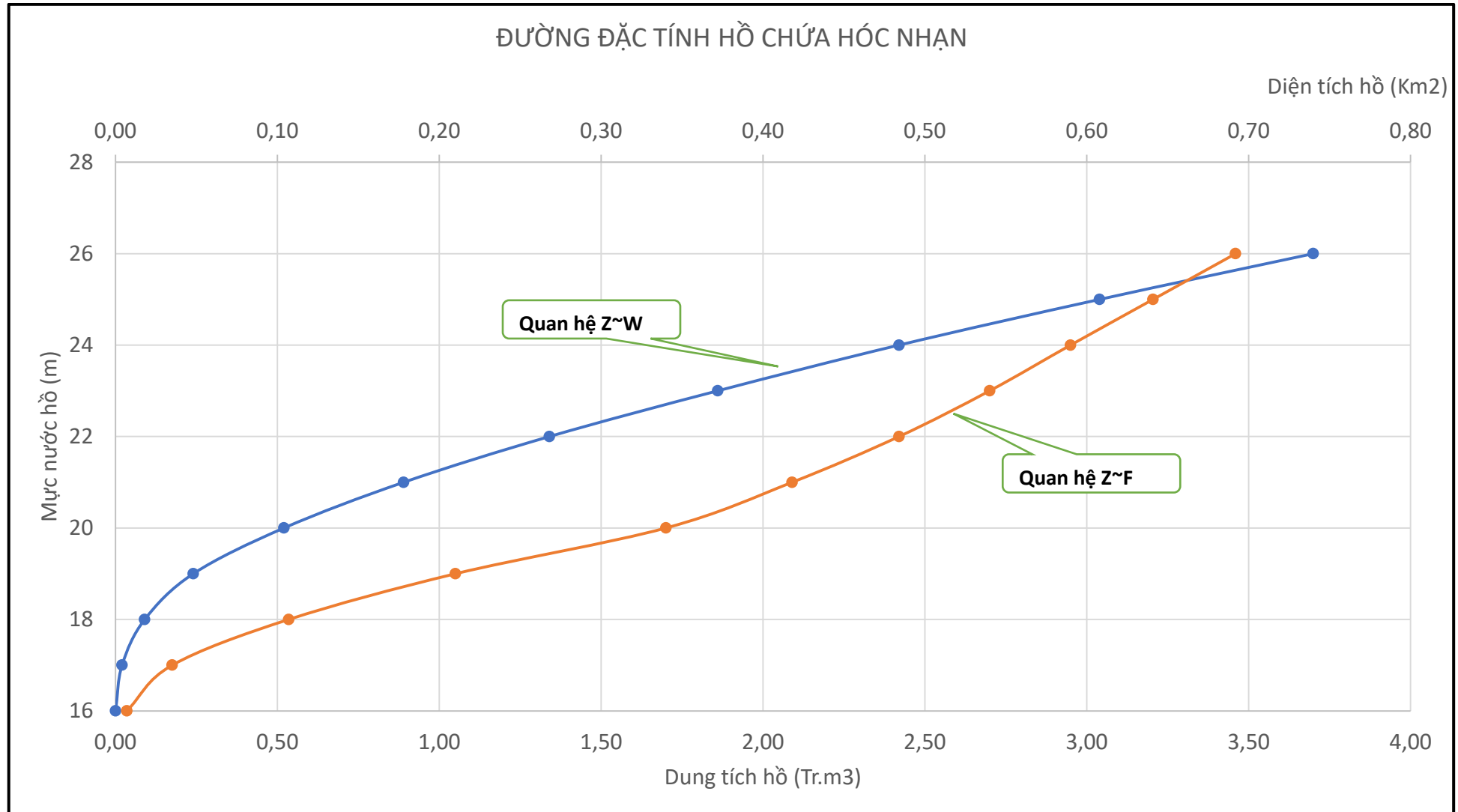
Hình PL8.1 Đường đặc tính hồ chứa nước Hóc Nhạn
