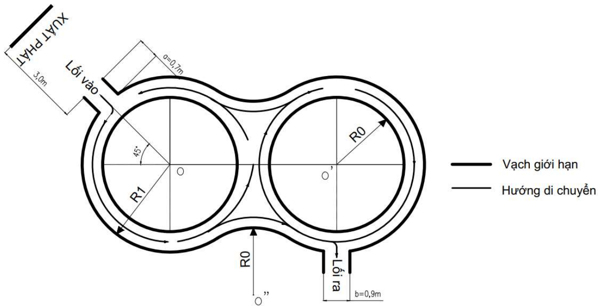
Hình 1: Hình bài sát hạch hình số 8
