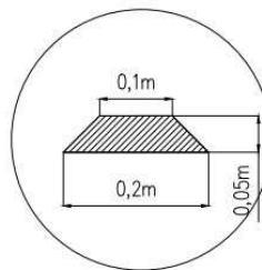
TIẾT DIỆN DẢI GỜ GHÈ HẠNG A1 - A
