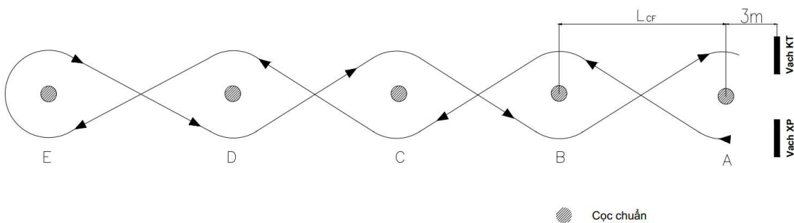
Hình 18: Hình bài sát hạch đi qua 05 cọc chuẩn hạng C1E, CE
