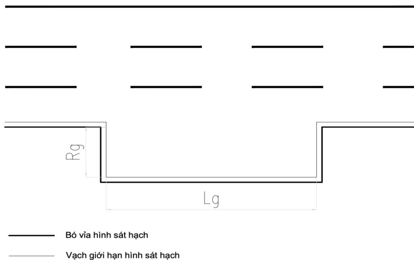
Hình 14: Hình bài sát hạch ghép xe ngang vào nơi đỗ đối với hạng C, D1, D2, D
