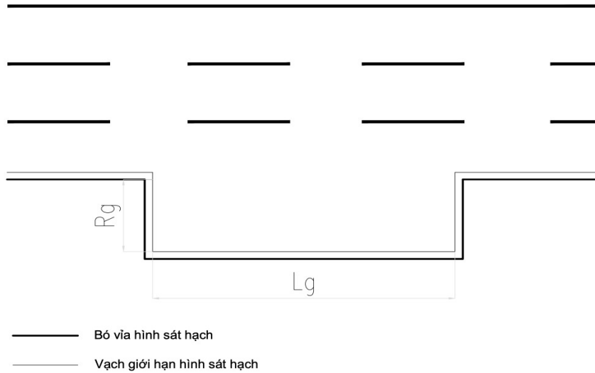
Hình 13: Hình bài sát hạch ghép xe ngang vào nơi đỗ đối với hạng B
